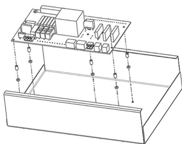
Przykładowy sposób montażu modułu we wnętrzu zabudowy.
