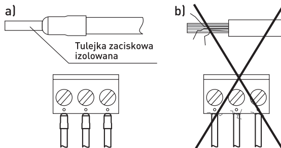
Zabezpieczanie końców przewodów: a) prawidłowe, b) nieprawidłowe.
