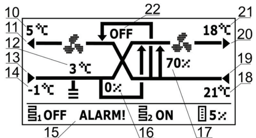
Ekran z wyświetlanym schematem automatyki
