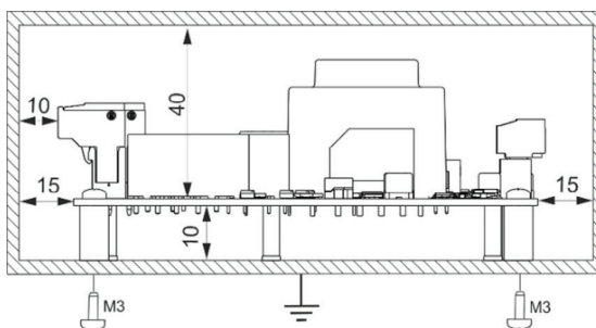
Przykładowy sposób montażu modułu we wnętrzu zabudowy.
